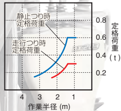
RX-203S CR 定格荷重 (標準アーム、0.06m 3 バケット付)
